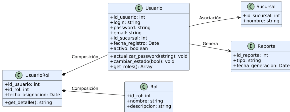
SIGA-Óptica - Diagrama de Clases (Usuarios y Roles)
