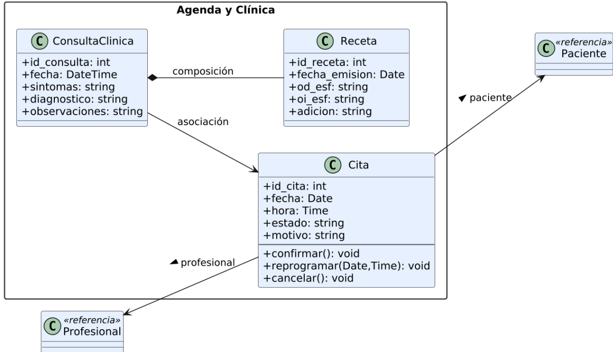
SIGA-Óptica - Diagrama de Clases (Agenda y Clínica)
